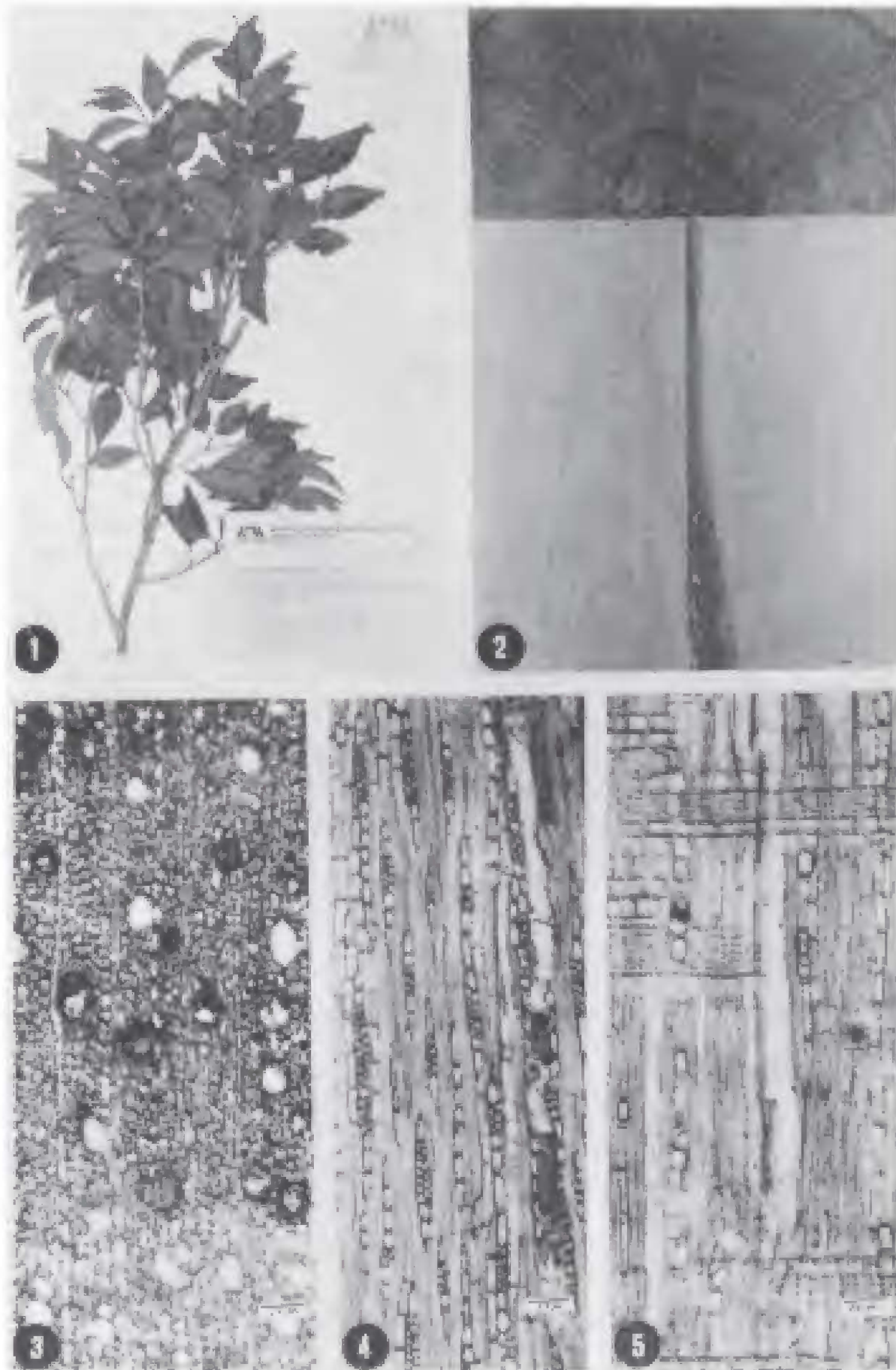
Figs. 1-5. Psidium sartorianum . 1. Muestra de herbario. 2. Tablillas de los tres cortes típicos: transversal (arriba), tangencial (izquierda) y radial (derecha). 3. Corte transversal. 4. Corte tangencial. 5. Corte radial.
